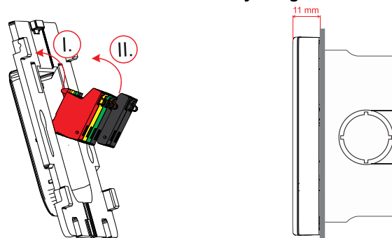
Rys. 3: Ilustracja częściowo zagłębionej instalacji
